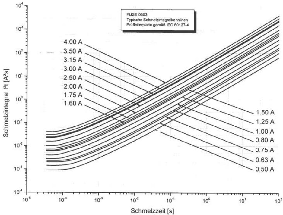
Typische I 2 t - t Kurven der FUSE 0603
